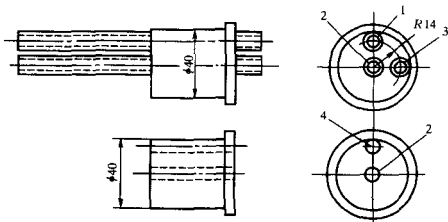
图 1 定位块示意图
