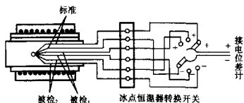
图1 检定时连接线路图
